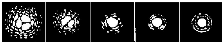
Рис. 5-3 Условия видимости напрямую влияют на качество изображения. На зарисовках изображен точечный объект (звезда) при очень плохой (слева) и идеальной (справа) видимости. Чаще всего атмосферные условия позволяют наблюдать изображения, переходные между этими противоположностями.
