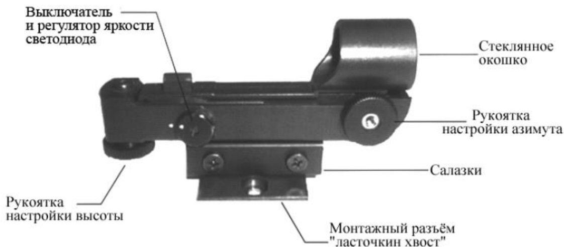
Рис. 3-3 Искатель Star Pointer
