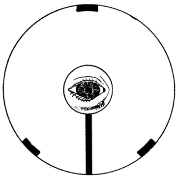
Вид в фокусирующий узел телескопа 114 LCM. Юстировка правильная.
