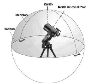
Рис. 4-3 Меридиан – это воображаемая линия на небосклоне, проходящая через Северный небесный полюс, зенит и Южный небесный полюс. С точки зрения наблюдателя, лицо которого обращено на север, меридиан начинается от северного горизонта и
